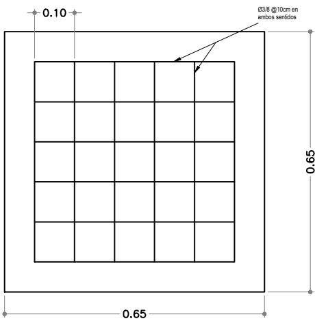
DETALLE ESTRUCTURAL
