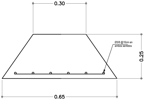
DETALLE ESTRUCTURAL
