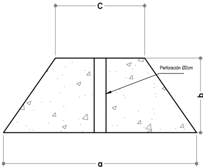
DETALLE DE ANCLA CONCRETO
