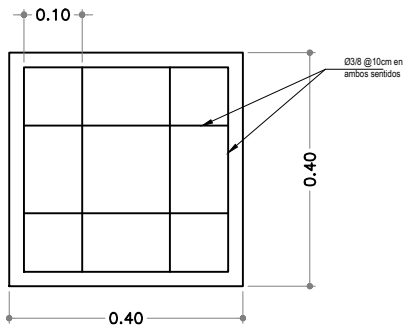
DETALLE ESTRUCTURAL
