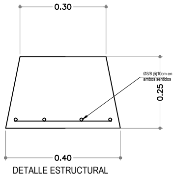
DETALLE ESTRUCTURAL
