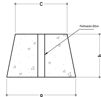
DETALLE DE ANCLA CONCRETO
